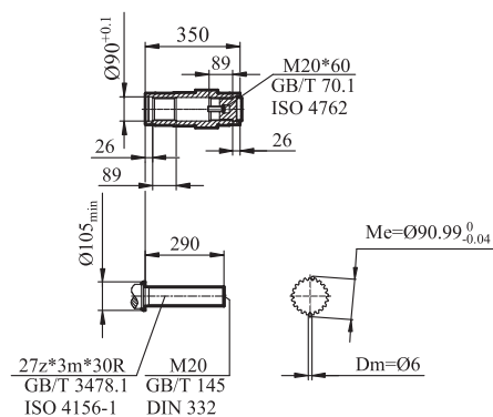
GFV/GFVZ/GFVF107输出轴
