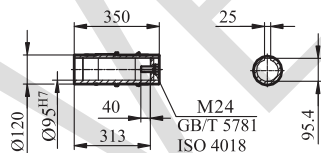
GFA/GFAZ/GFAF107输出轴
