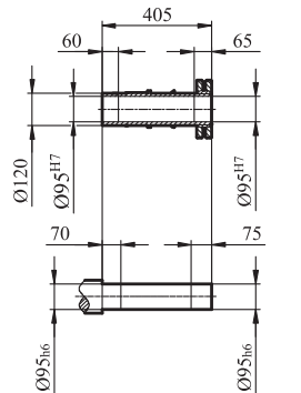
GFH/GFHZ/GFHF107输出轴
